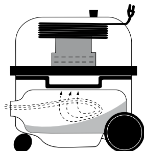
Ketelmodel
